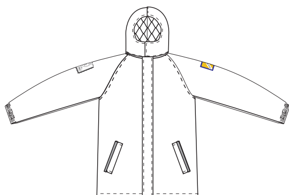
- COLOCADO EN BOLSILLO, DELANTERO O ESPALDA A MODO DE VIVO CON R1A
