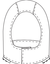
- CAPUCHA DESMONTABLE CON CIERRE PVC O METALICO. AJUSTE DE BROCHE PVC O METALICO. CON O SIN AJUSTE DE CORDON ELASTICO
